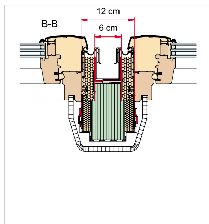
Kombinace pomocné krokve EKS s napojením na systémové ostění Roto ZIN
